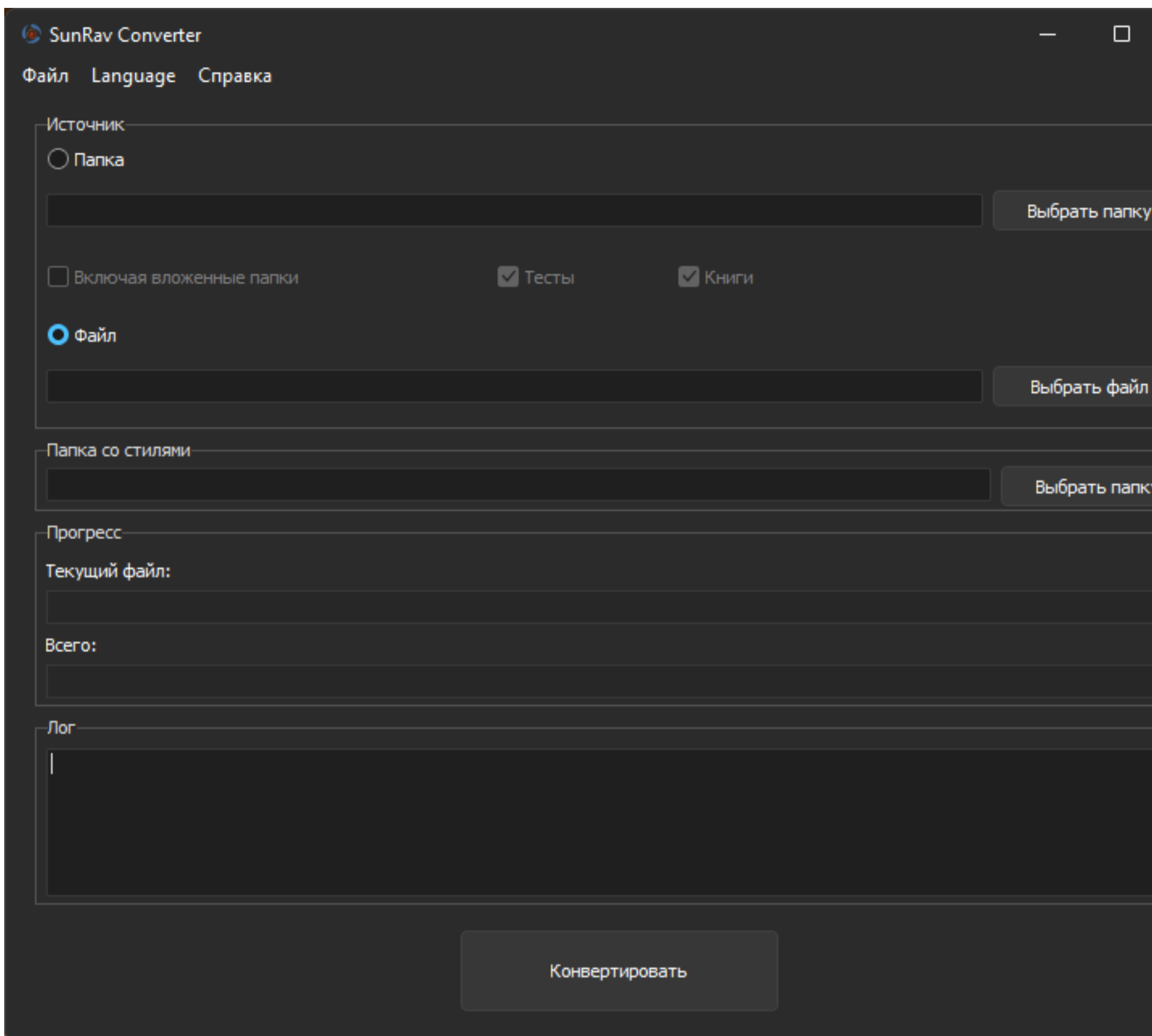
Рис. 1. Главное окно программы SunRav Converter
